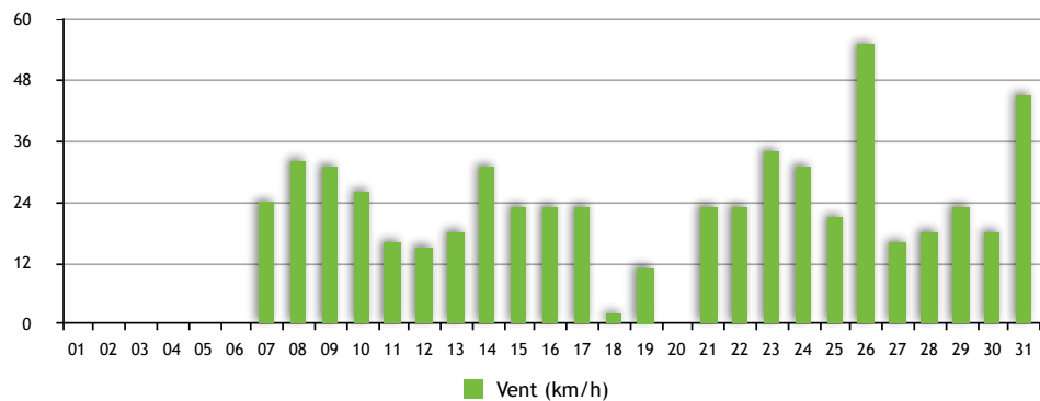
Vent
