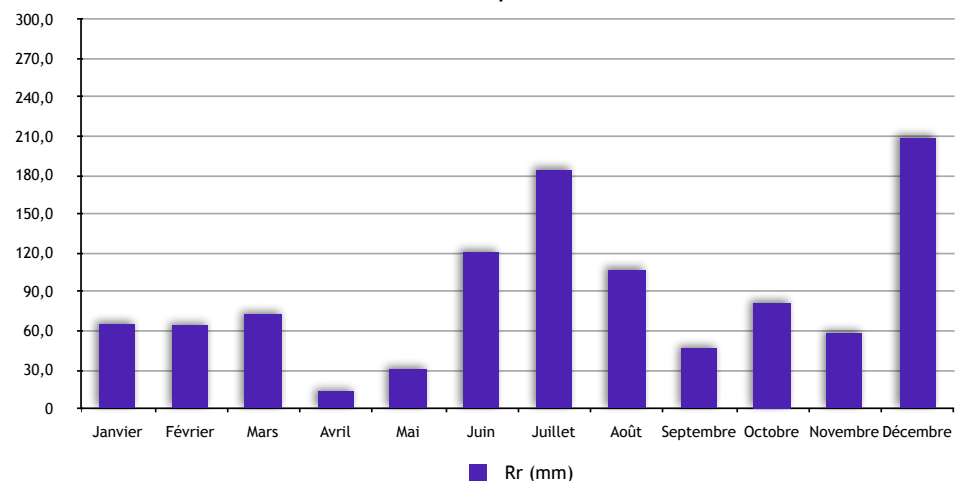
Précipitations
