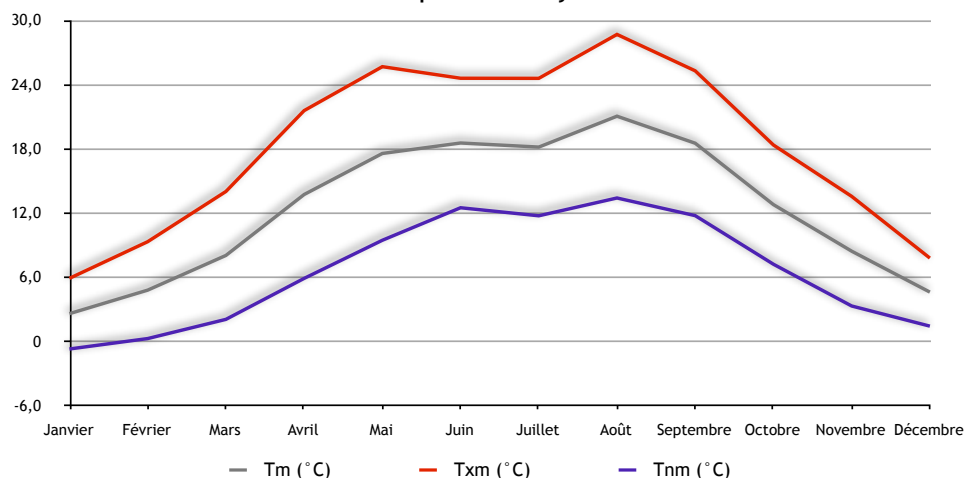
Températures moyenne
