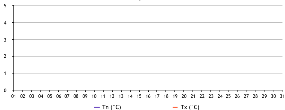
Températures
