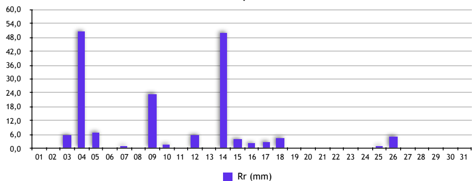
Précipitations
