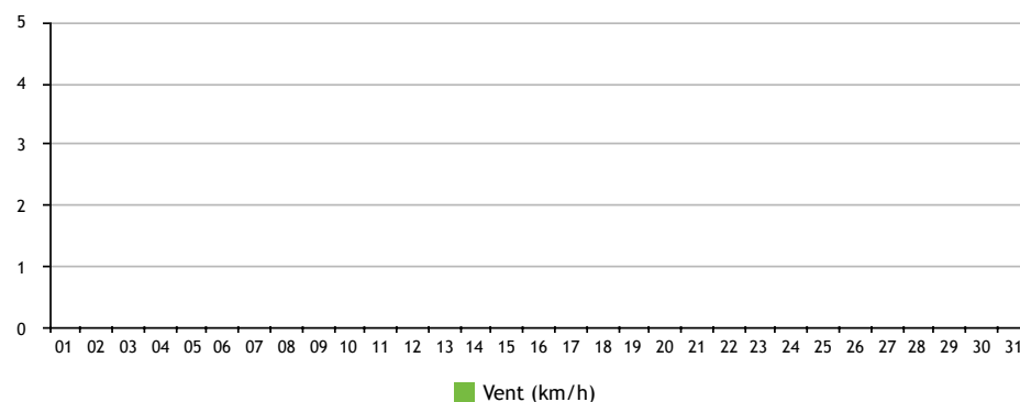
Vent
