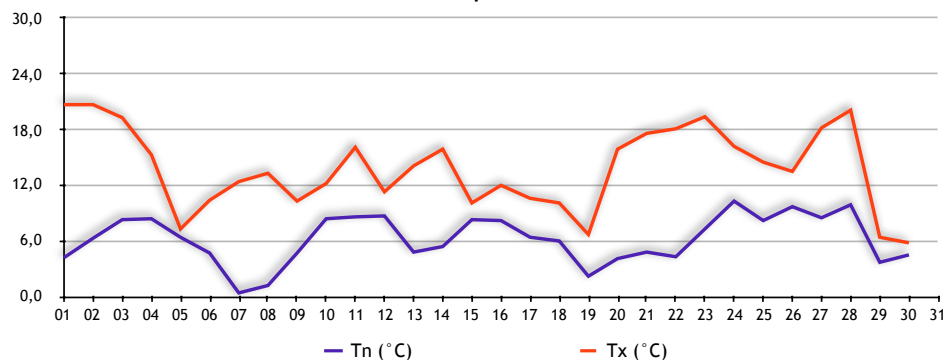
Températures
