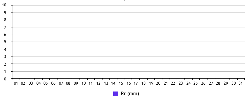
Précipitations
