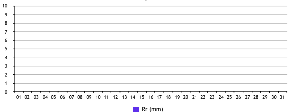
Précipitations
